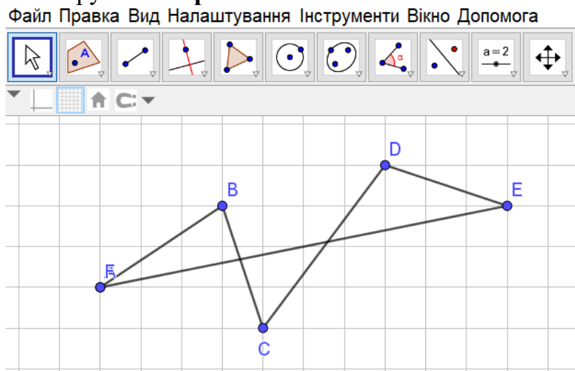
Рис.1.18 Замкнена ламана
