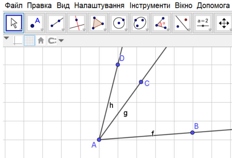
Рис.1.14 Три кути
