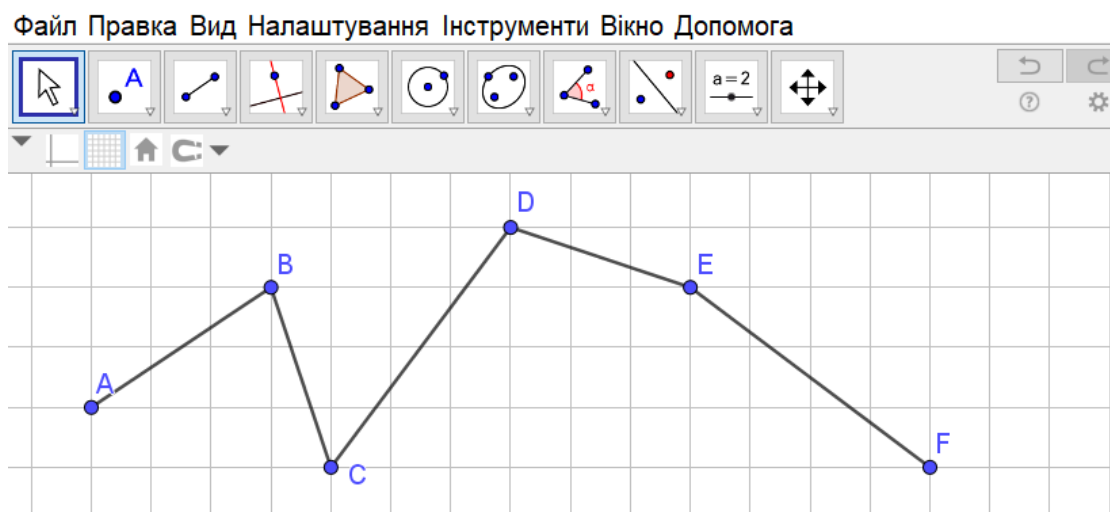
Рис.1.17 Ламана
