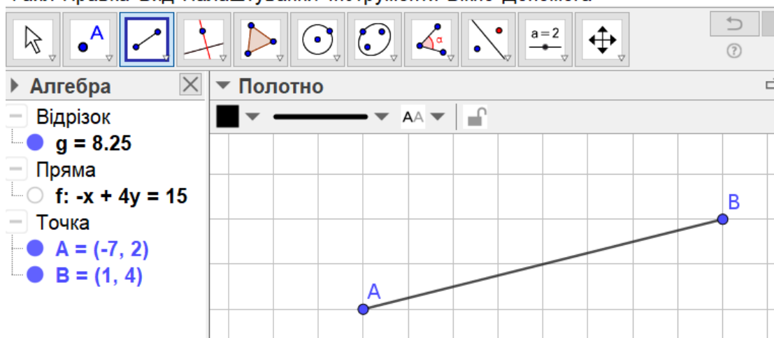
Рис.1.10 Відрізок AB
