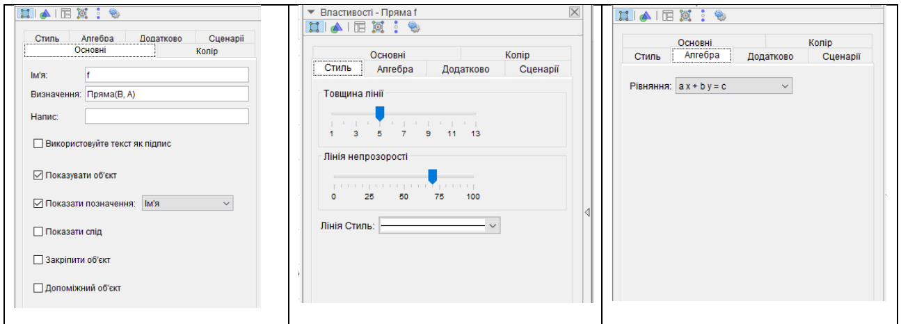
Рис.1.8 Властивості прямої
