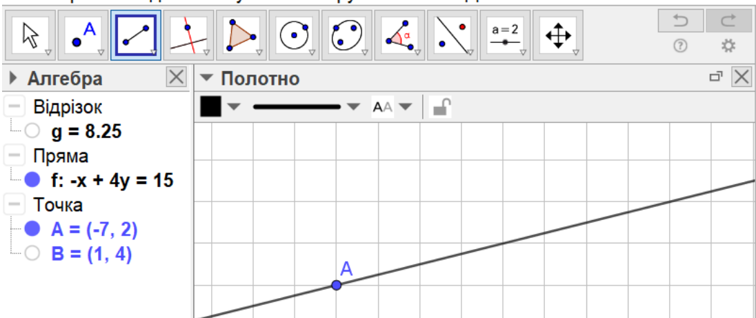
Рис.1.11 Поділ прямої на два промені
