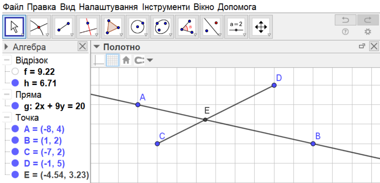
Рис.1.12 Розбиття площини на півплощини
