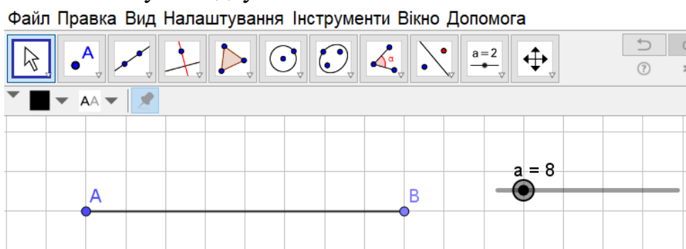
Рис.1.22 Відрізок, довжину якого можна змінювати повзунком
