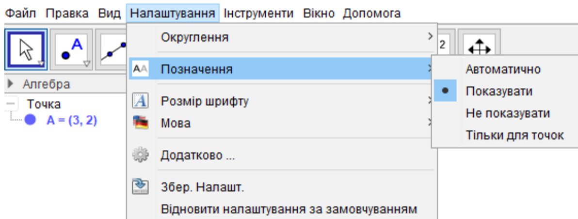
Рис.1.3 Меню Налаштування
