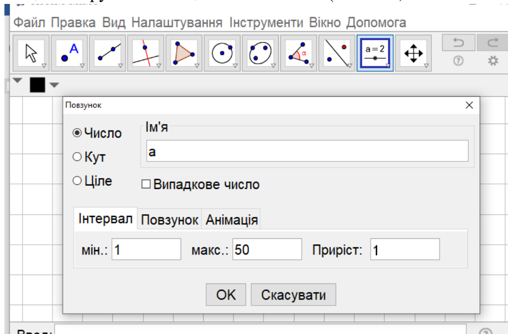
Рис.1.21 Побудова повзунків
