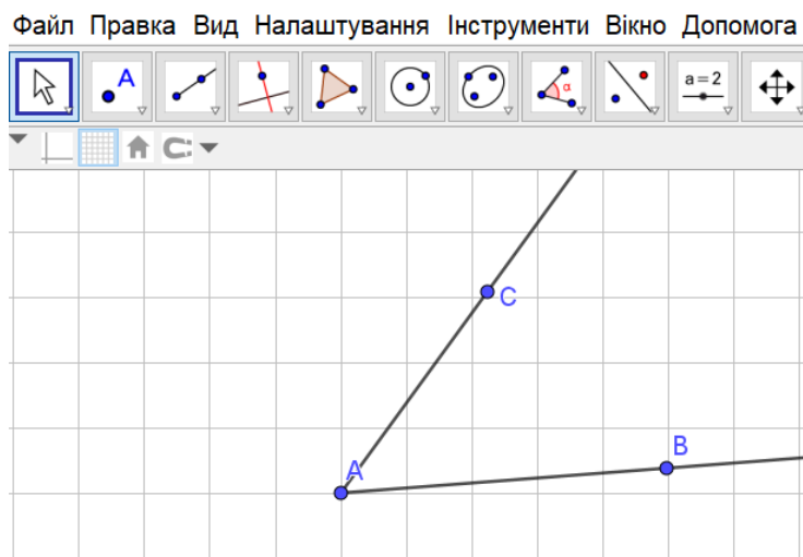
Рис.1.13 Кут
