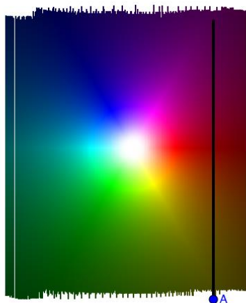
Figura 5. Traza del escáner para la función f(z)= 1/z .
