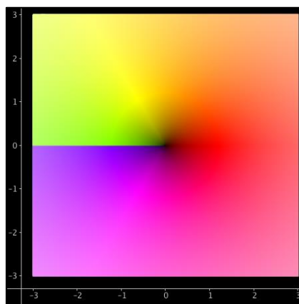
Figura 3. La función f(z)=z^{1/2} .
